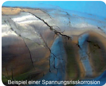
Beispiel einer Spannungsrisskorrosion
